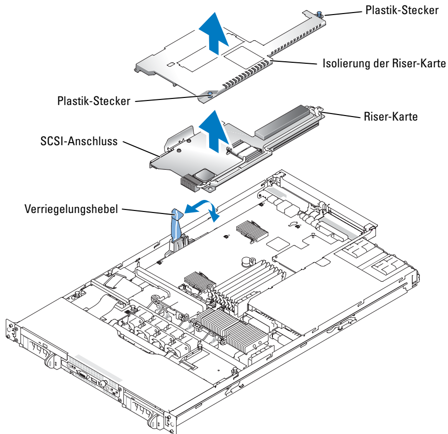
Abbildung 1-1. Riser-Karte installieren und entfernen
