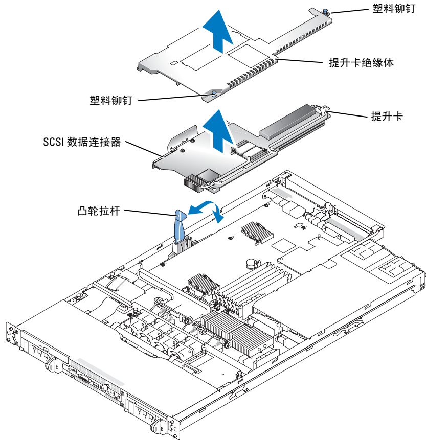
图 1-1. 装卸提升卡
