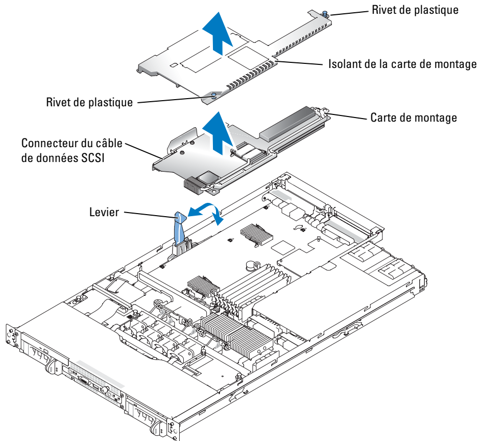
Figure 1-1. Installation et retrait de la carte de montage
