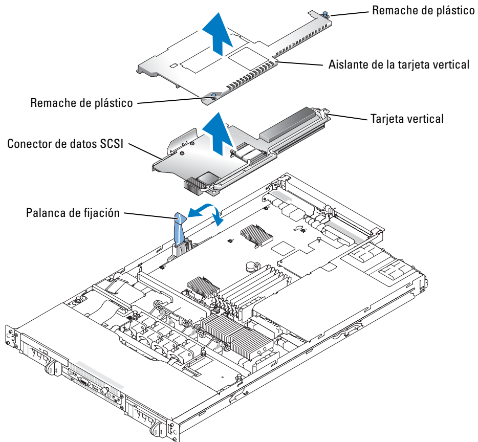
Figura 1-1. Instalación y extracción de la tarjeta vertical
