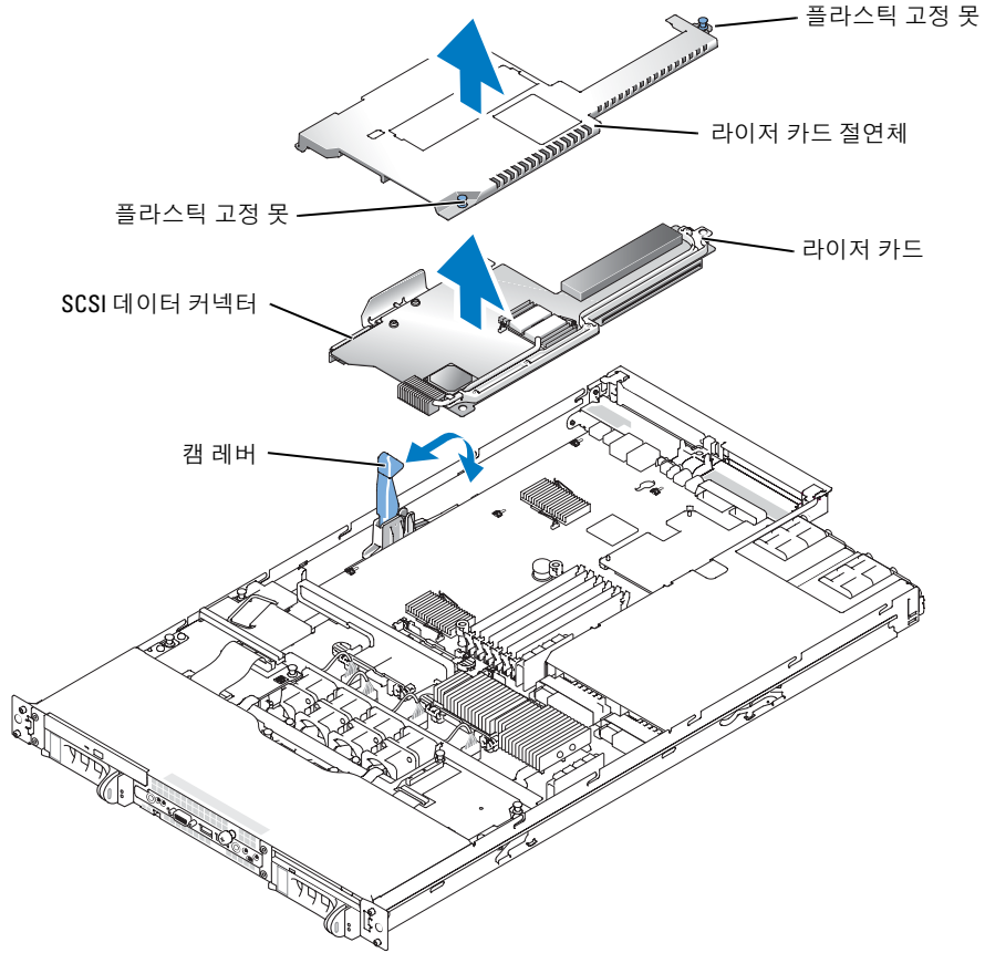
그림 1-1. 라이저 카드 설치 및 분리
