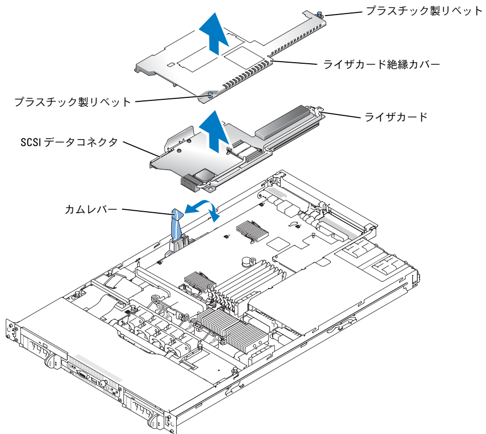
図 1-1 ライザカードの取り付けと取り外し
